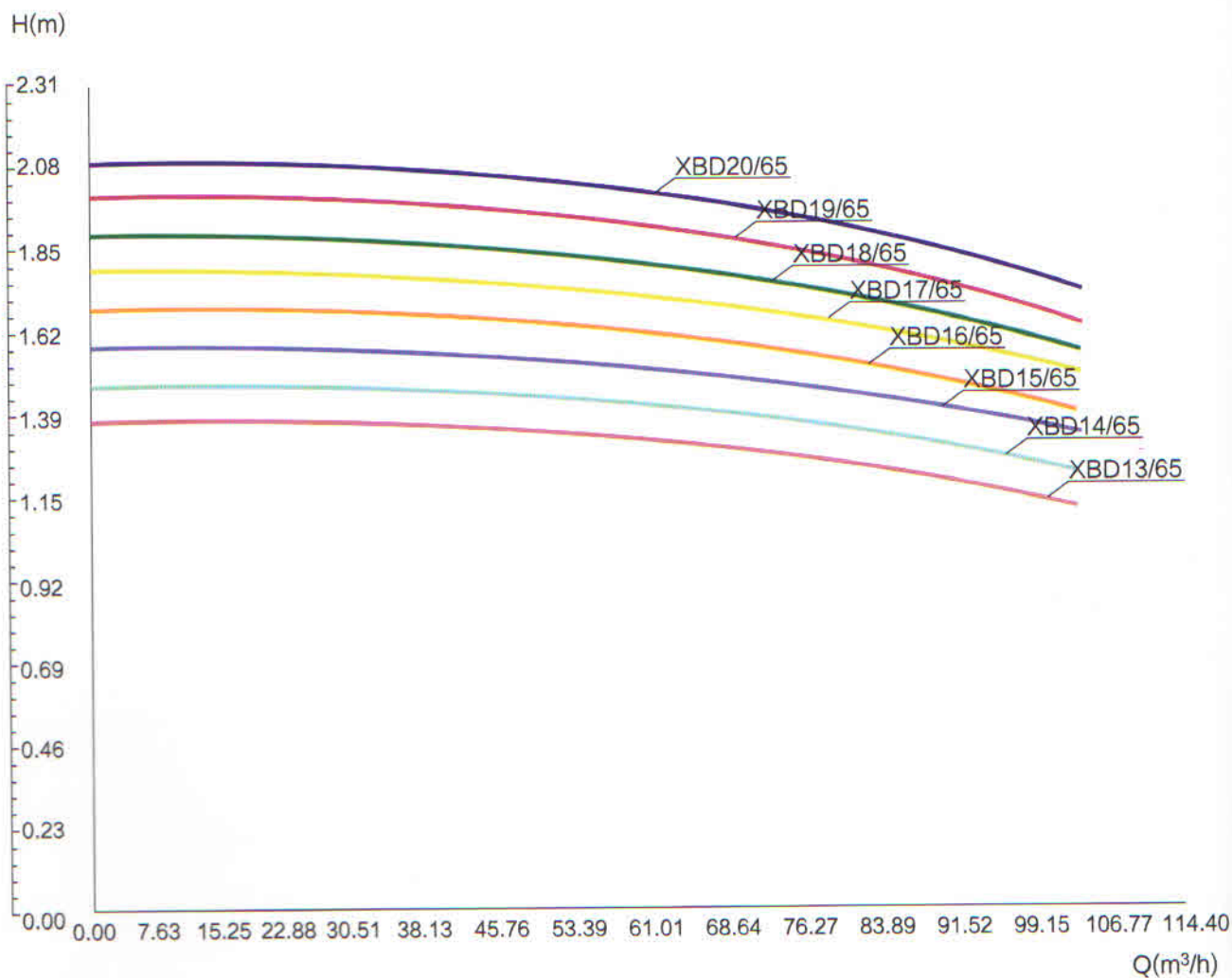
Q/H 性能曲线
